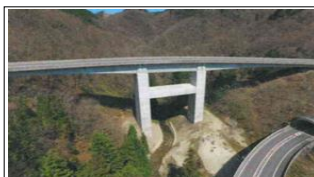
新平家橋工事 (橋梁耐震)
